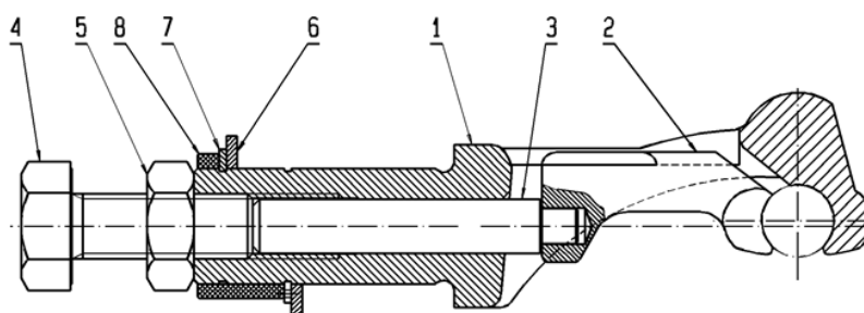
Слика 1. Фиксна стезаљка
