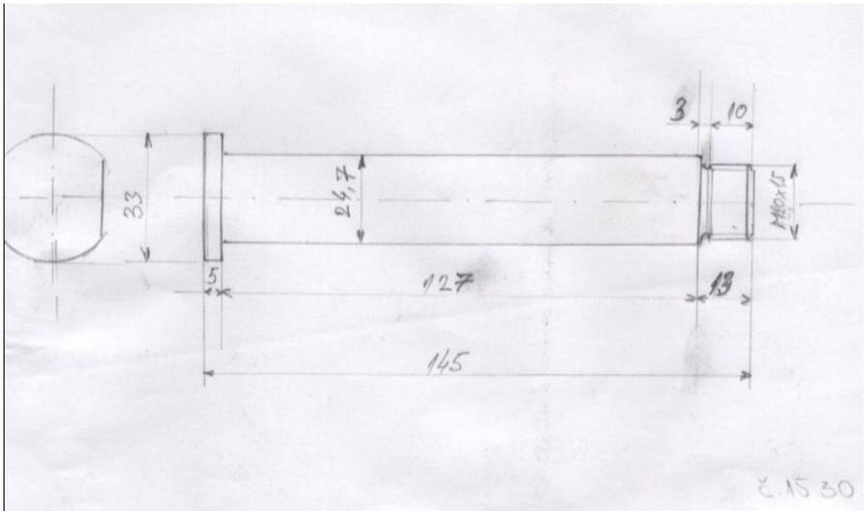
Осовина редни бр. 12 из табеле
