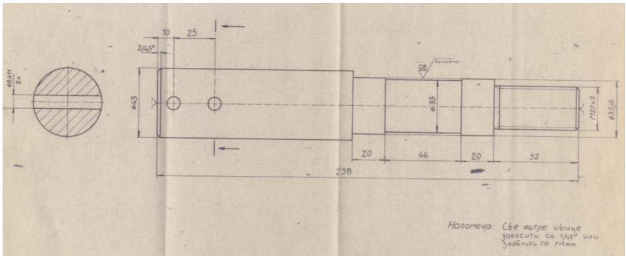
Осовина редни бр. 12 из табеле
