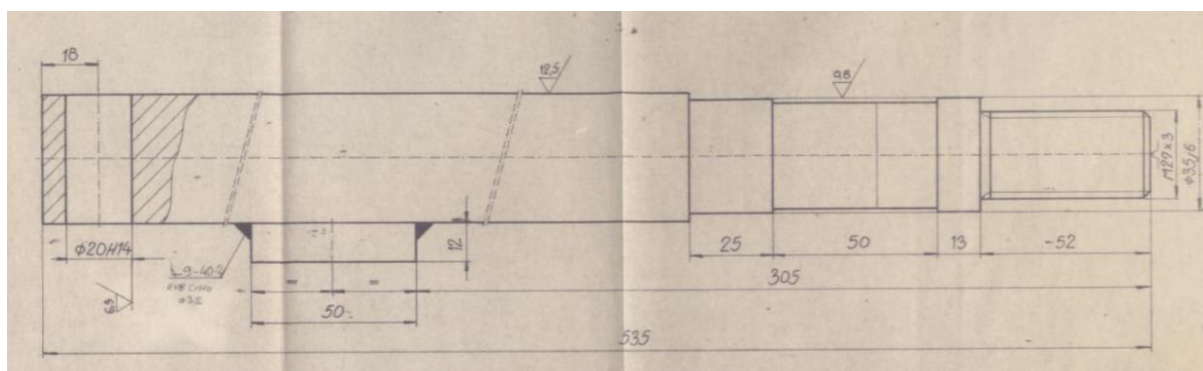
Осовина редни бр. 14 из табеле
