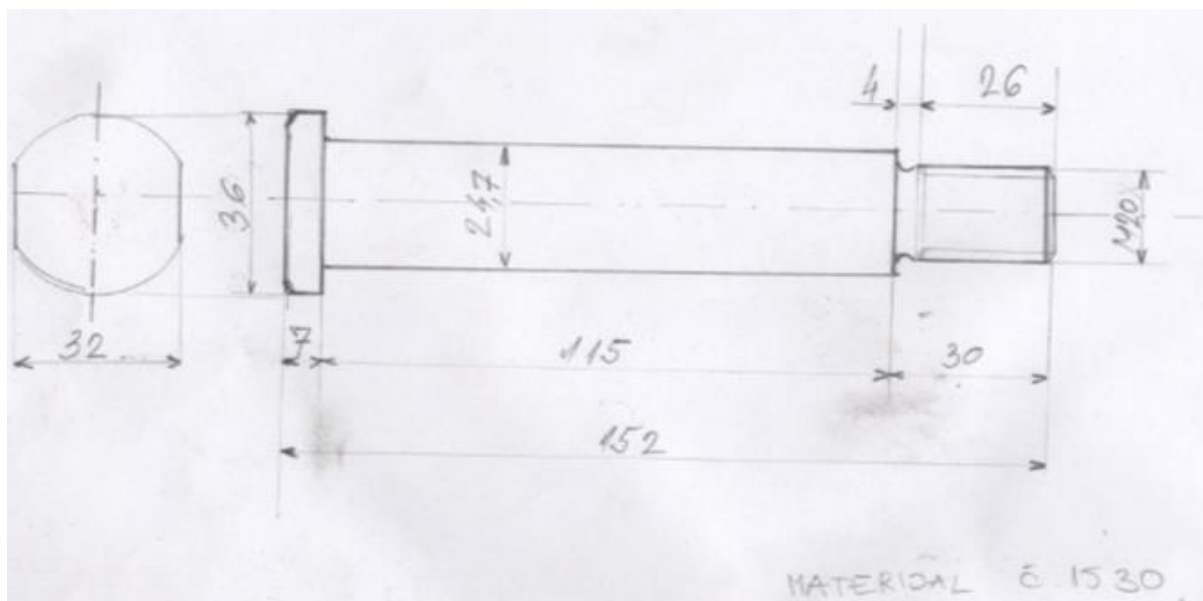
Осовина редни бр. 13 из табеле
