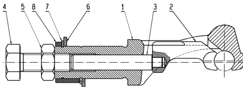
Слика 1. Фиксна стезаљка Doppelmayr
