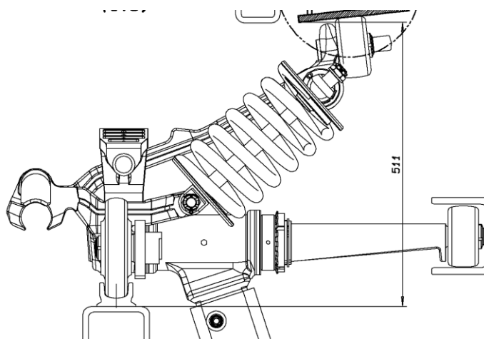
Слика 2. Расклопива стезаљка Pomagalski и Lajtner
